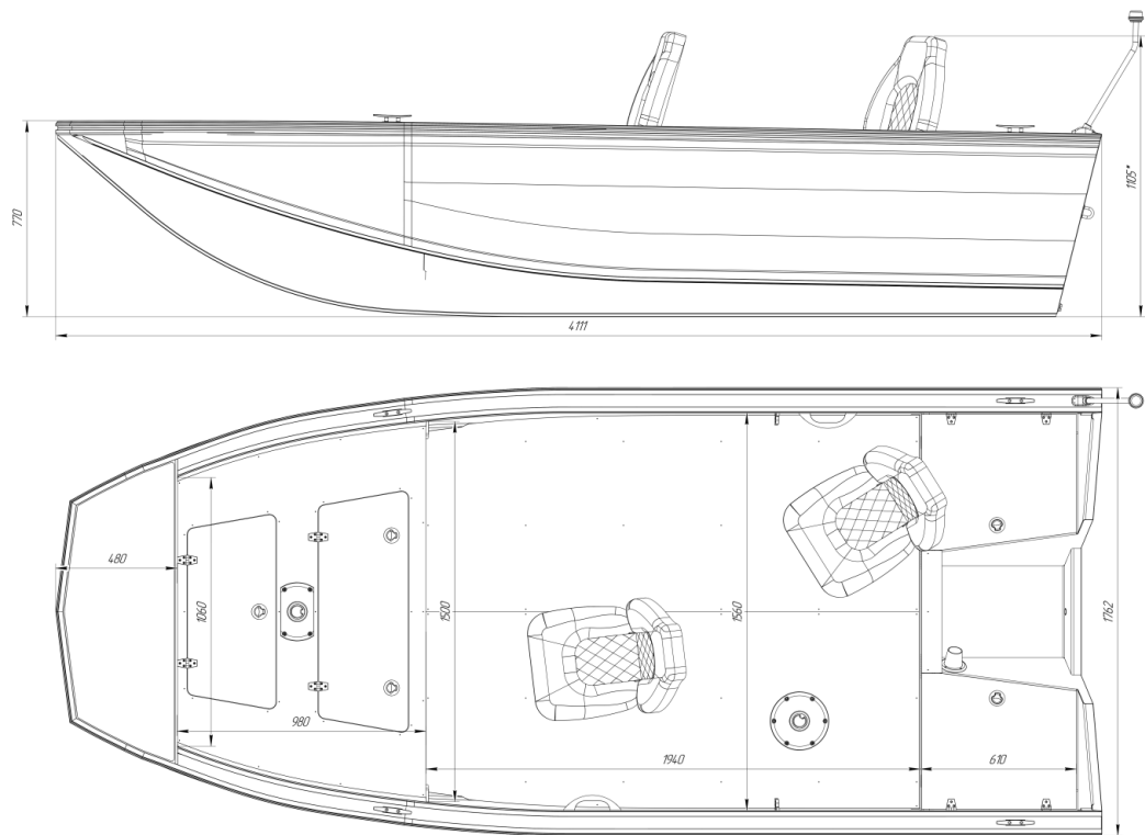
VIZION 410 Motorboat Diagram
